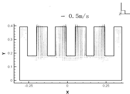
图 1 Z =0.25 电解槽截面的流场图
