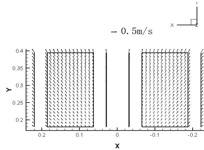
图 2 阳极流场分布图
