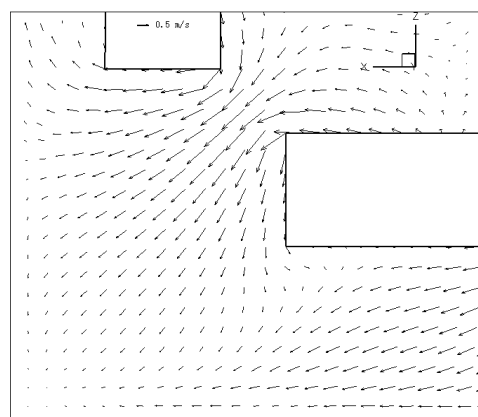
图 4 电解槽的上表面流场局部放大图
