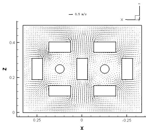
图 3 电解槽的上表面流场分布图
